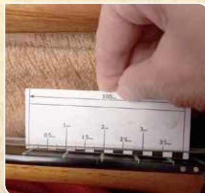
15. Comprobación de altura de cuerdas
